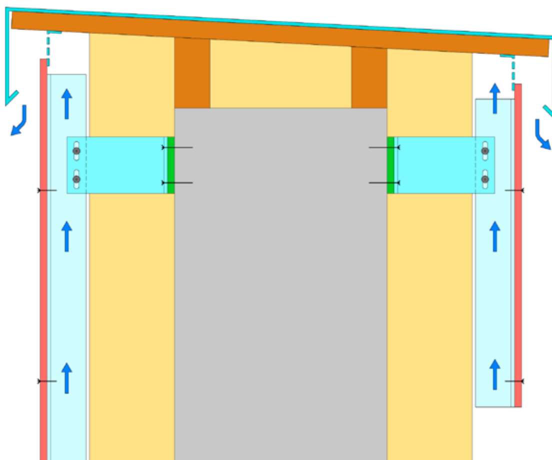
Abbildung 11 Oberer Abschluss
