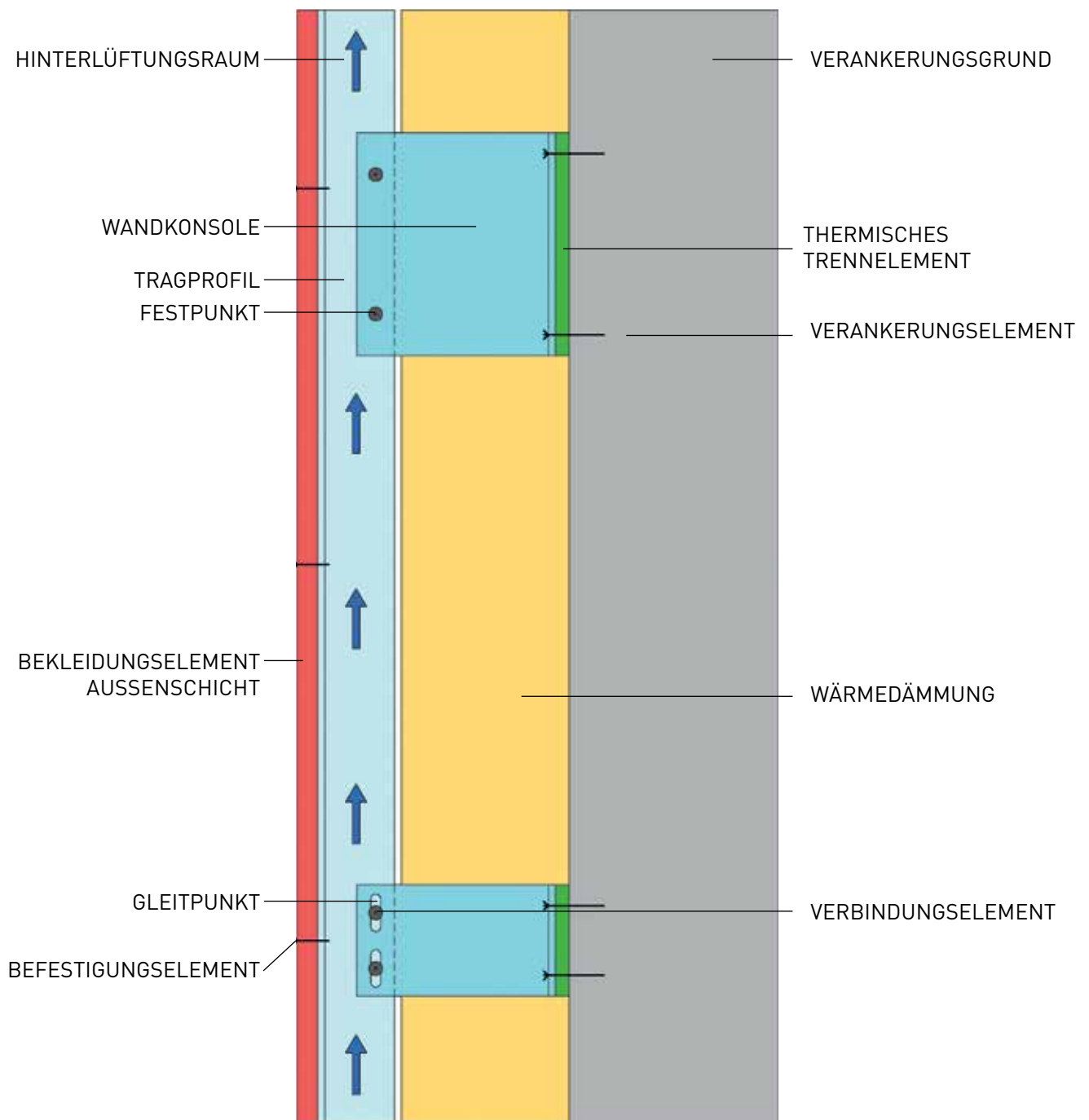
Abbildung 1 Begriffserklärung
